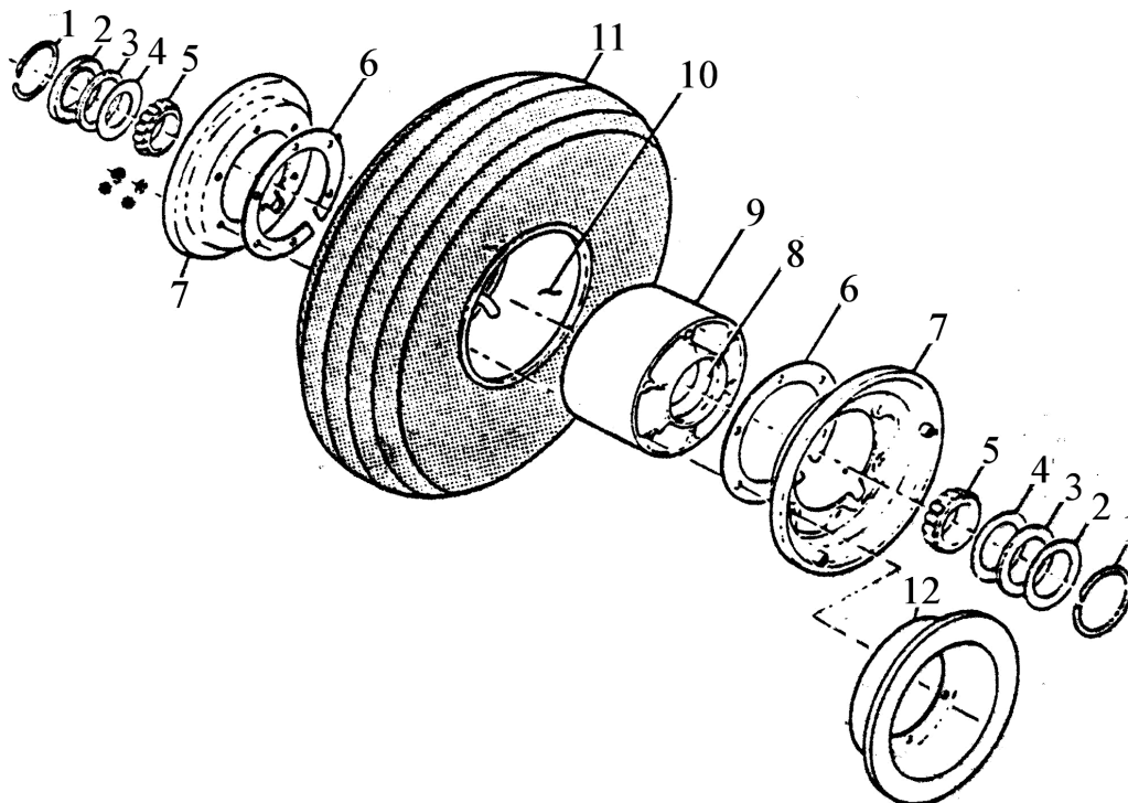
Rysunek 2. Budowa koła
