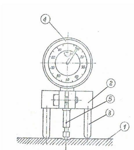
Rys. 1. Pomiar głębokości wgniecia
