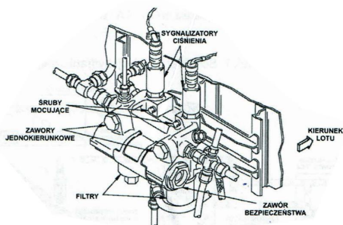
Rys. 29.15 Moduł ciśnienia
