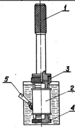
Rys. 04-03.1. Uchwyt do przemywania elementów filtrujących: 1 – rękojeść; 2 – element filtrujący; 3 – łącznik; 4 – korek; 5 - pędzel
