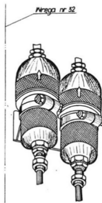
Rys. 04-03.3. Zamocowanie filtrów w stateczniku pionowym.
