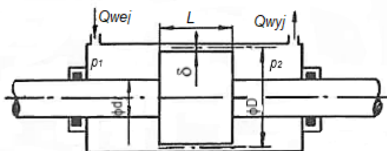
Rys. 1. Geometria elementów ruchomych
