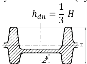
Rysunek 3. Prawidłowe położenie denka względem powierzchni podziału matryc
