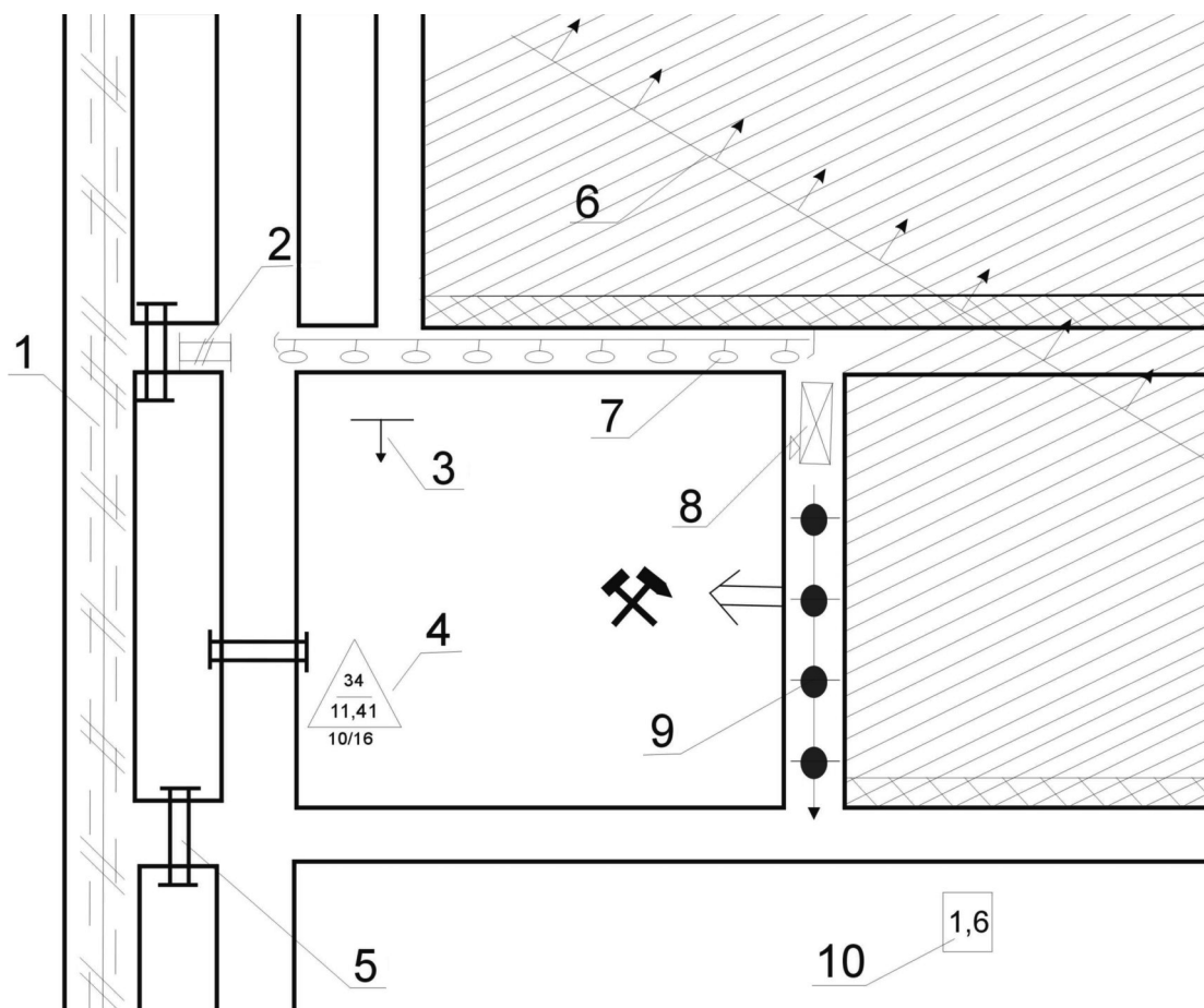
Rysunek 1. Wycinek mapy pokładowej
