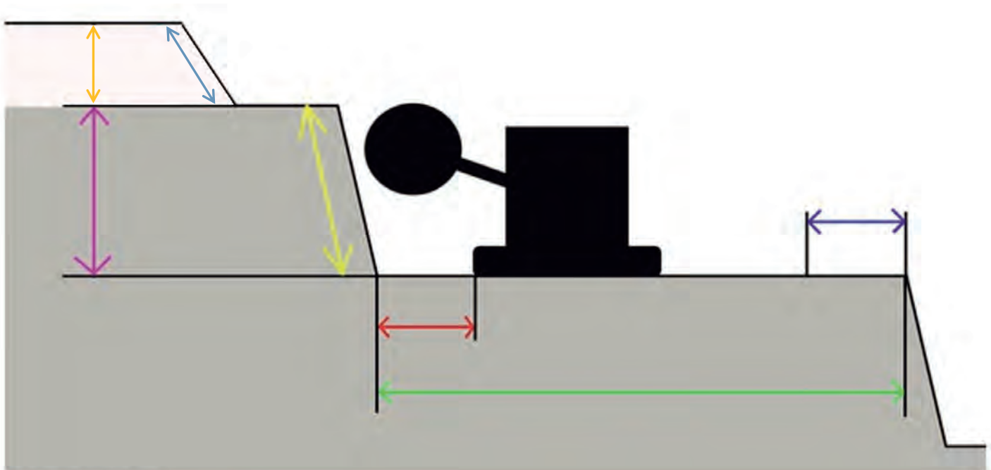
Rysunek Profil wyrobiska
