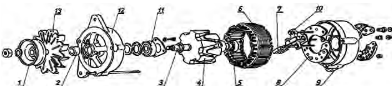
Rysunek 2. Alternator z rozłożonymi elementami.
