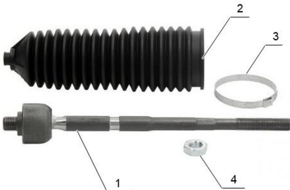
Rys. 3. Elementy zestawu naprawczego drążka kierowniczego Fiat 500C
