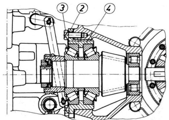
Rysunek 1. Wymontowanie wałka atakującego
