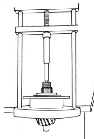
Rysunek 6. Wyciskanie wałka atakującego z obudowy łożysk
