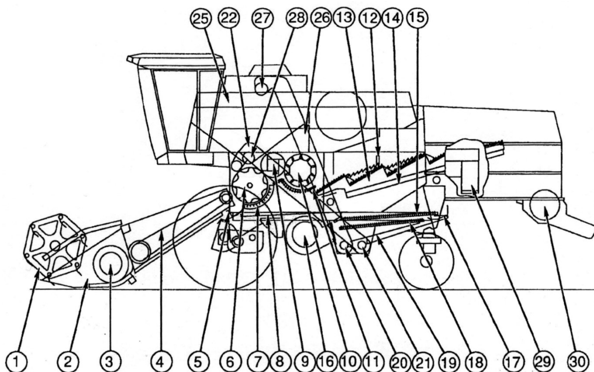
Rysunek 1: Ogólny schemat kombajnu
