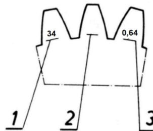
Rysunek 3. Oznakowanie czola zębów wałka atakującego
