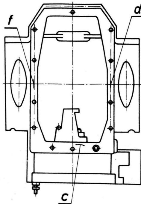
Rysunek 4. Oznakowanie korpusu tylnego mostu c, d, f – miejsca oznakowania (umieszczenia) odchyłek wymiarów c, d, f . c = - 0,27 mm
