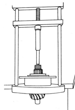
Rysunek 6. Wyciskanie wałka atakującego z obudowy łożysk
