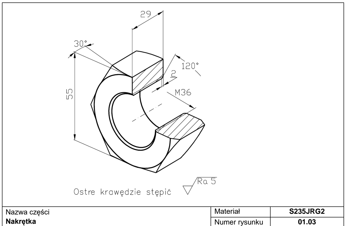
Rysunek 1. Nakrętka
