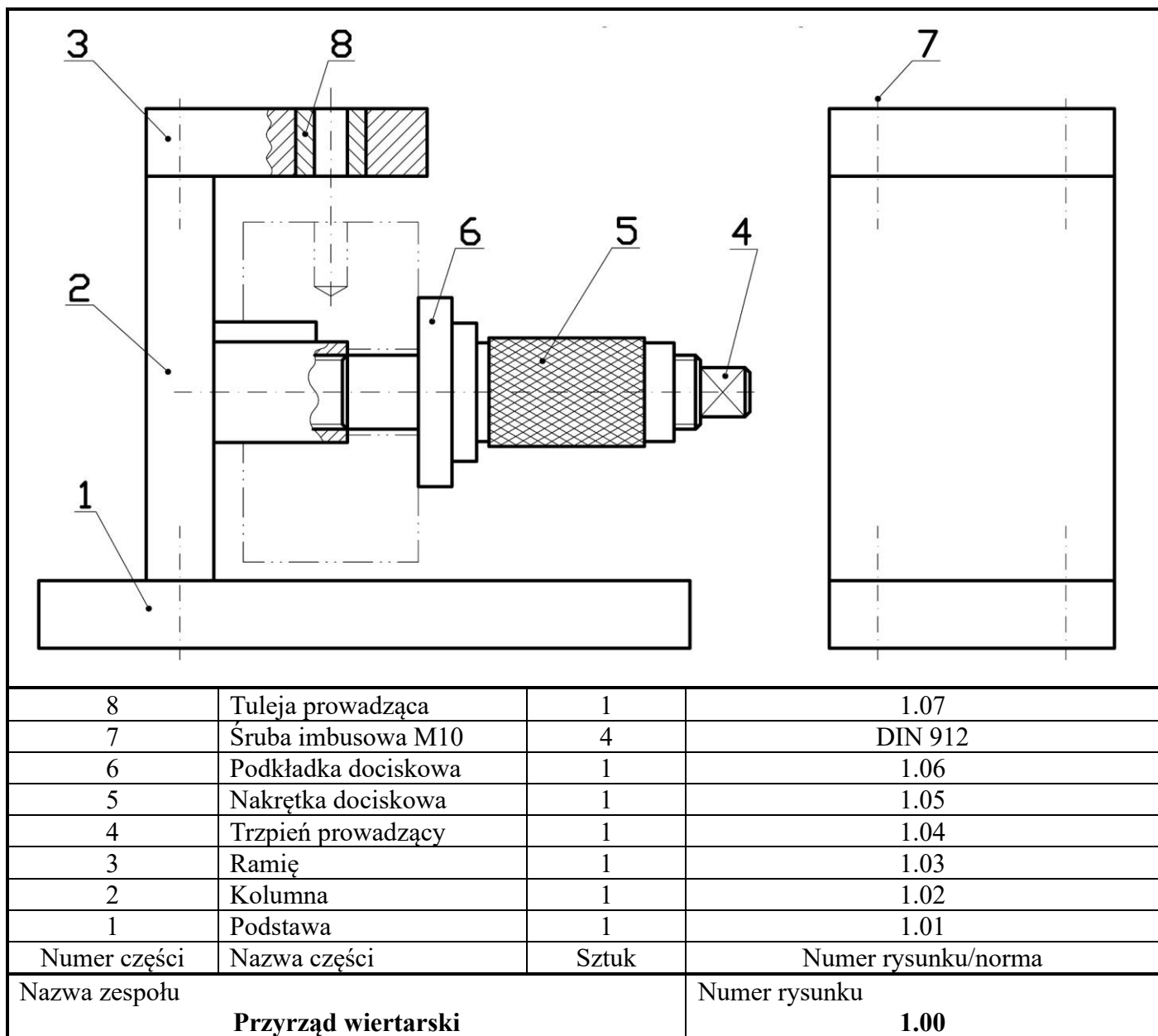
Rysunek 1.00. Przyrząd wiertarski
