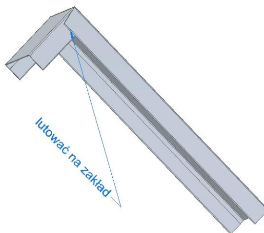
Rysunek 2. Rozwinięcie i widok wspornika daszka pojemnika
