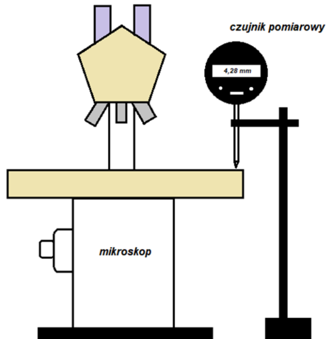
Rys.1 Schemat układu pomiarowego
