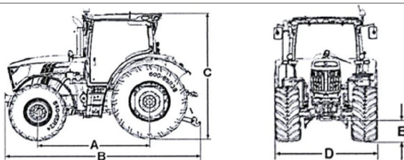
Fragment z instrukcji obsługi ciągników John Deere - dane techniczne (wymiaru podano w mm.)
