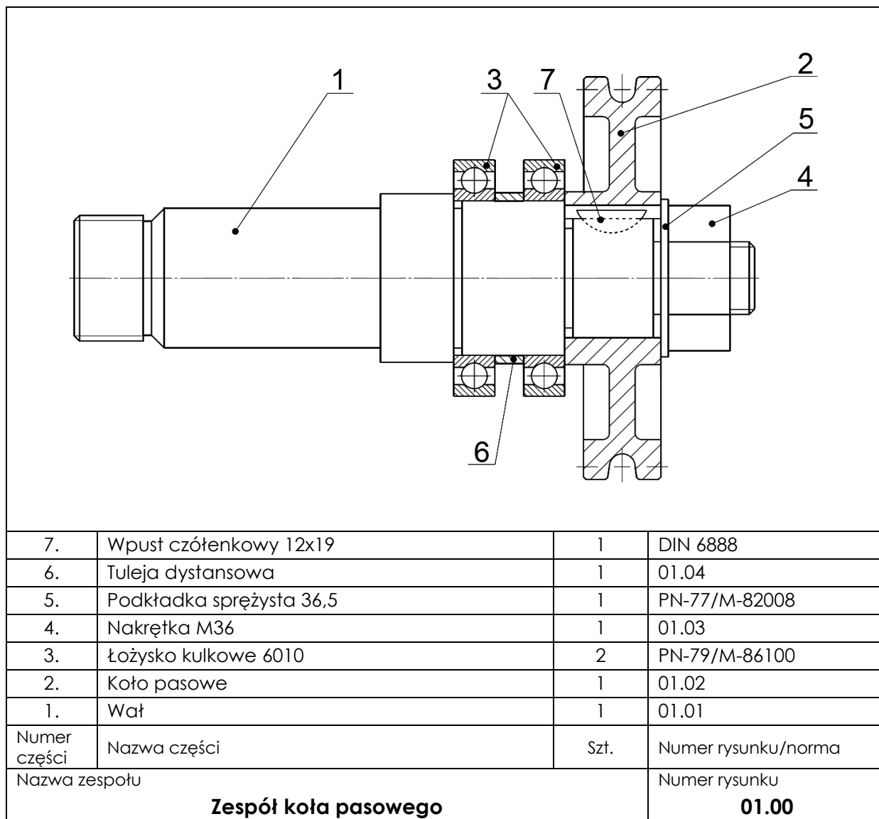
Rysunek 2. Zespół koła pasowego
