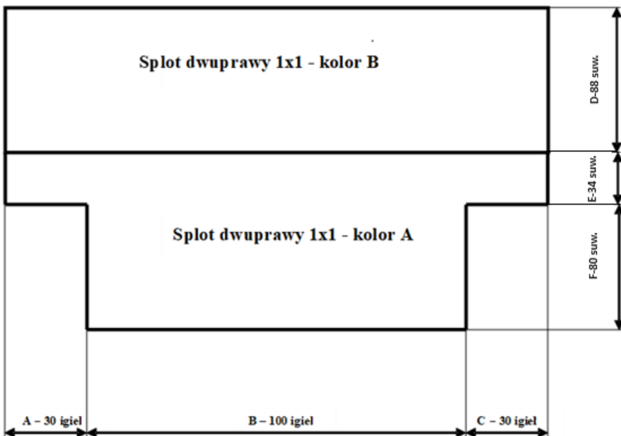
Rysunek 1. Wyrobu dzianego typu „szalik –golf”
