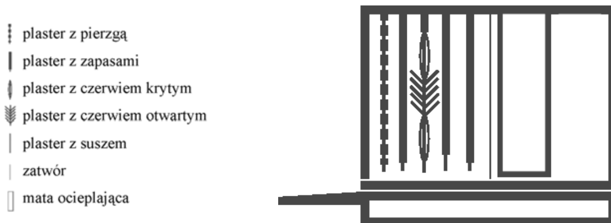
Rysunek. Ułożenie ramek w gnieździe
