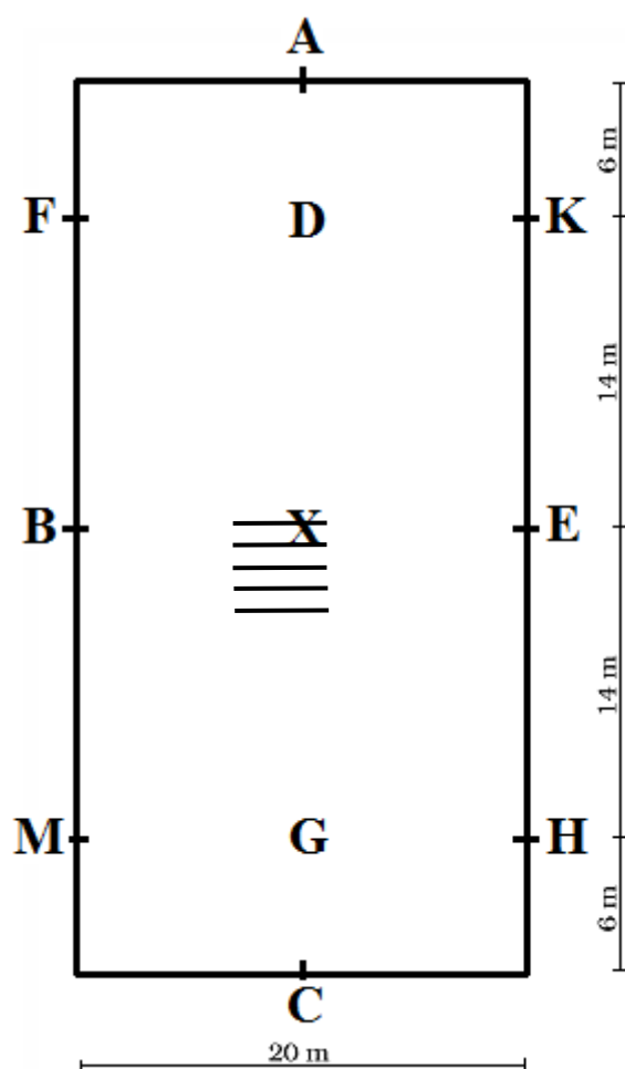
Schemat czworoboku/ujeżdżalni
