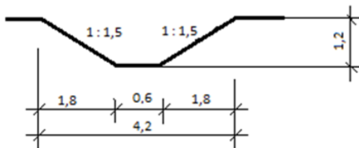
Rysunek 1. Przekrój poprzeczny rowu
