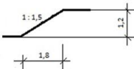
Rysunek 3. Skarpa rowu do wymiarowania
