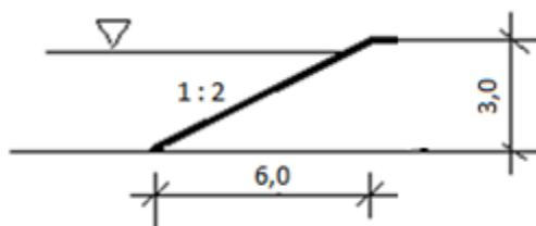
Skarpa odwodna wału
