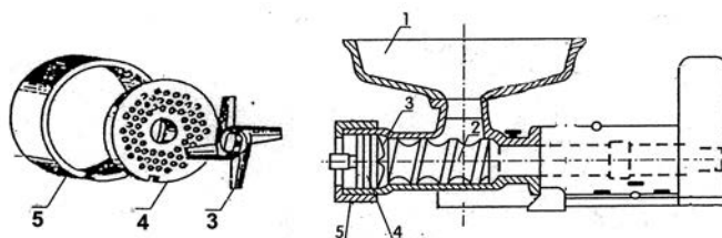
1 – misa załadownicza, 2 – ślimak, 3 – nóż, 4 – siatka, 5 – pierścień dociskający
