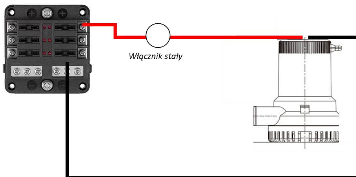
Rysunek 5. Uproszczony schemat elektryczny
