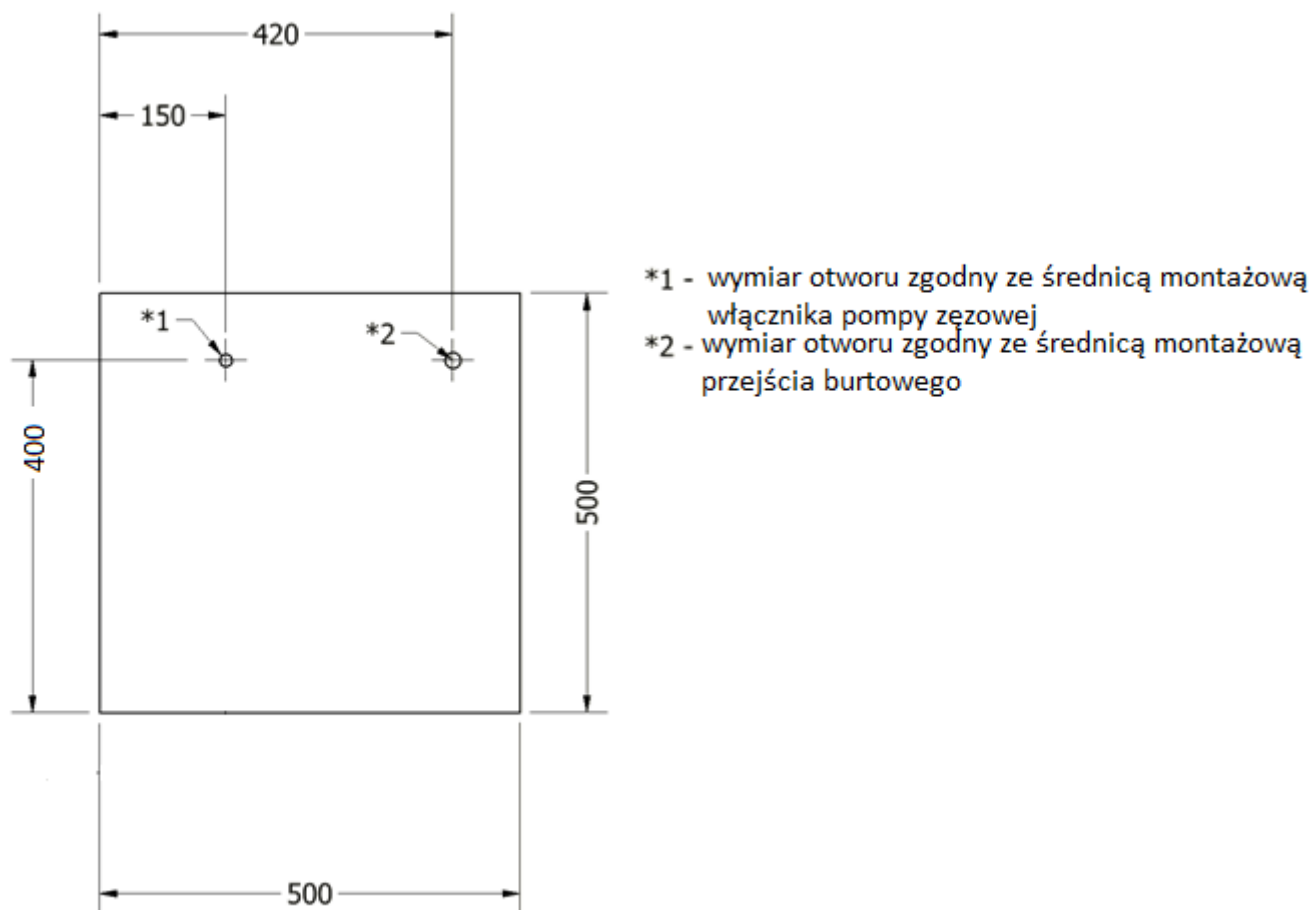
Rysunek 2. Ścianka montażowa
