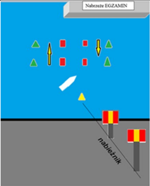
Załącznik 1. Plan toru wodnego
