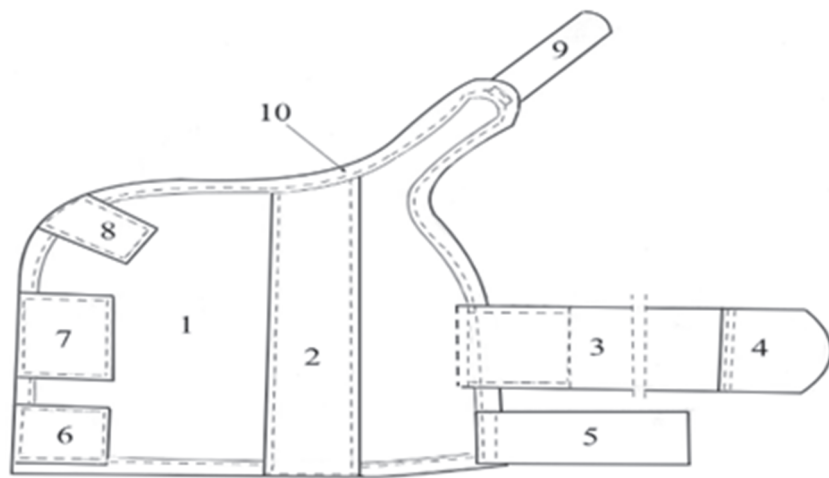
Rys.1 Stabilizator w rozłożeniu - wierzch
